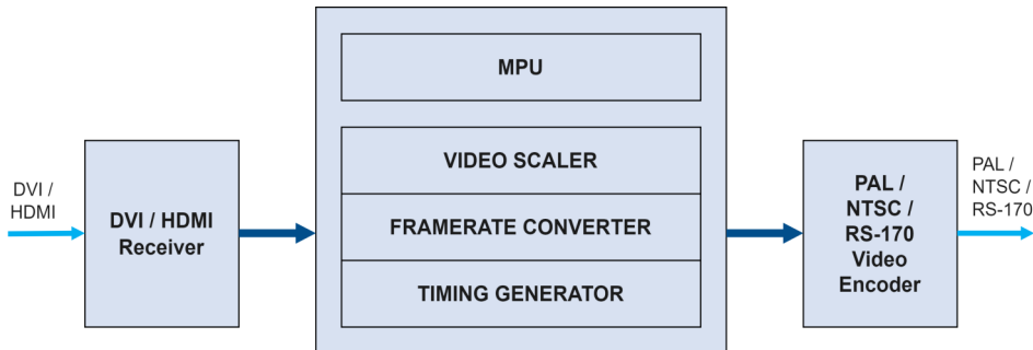
HDMI2COMP-IS-OEM Functional Diagram
